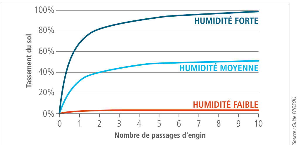
Représentation schématique du tassement du sol forestier en fonction du nombre de passages d'engin et de l'humidité du sol
